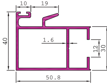
20835 0.904 kg/m
