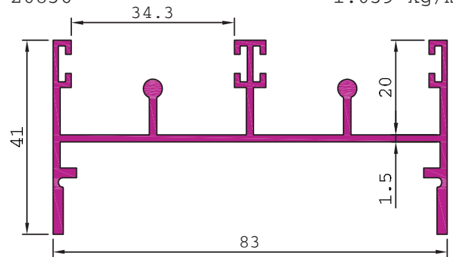
20836 1.039 kg/m
