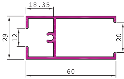
20859 0.775 kg/m
