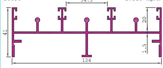
21175 2.298 kg/m
