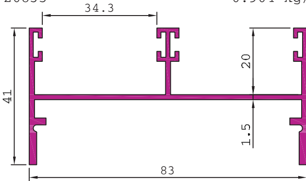
20835 0.904 kg/m
