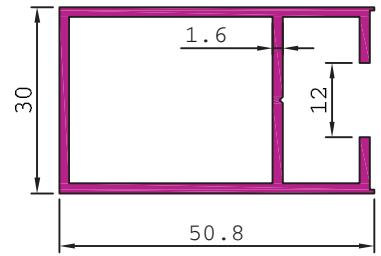
20553 0.731 kg/m
