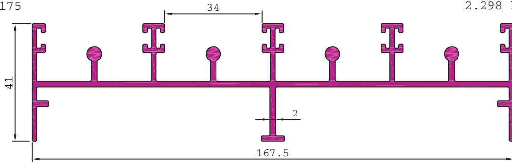
21176 1.745 kg/m
